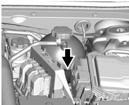
Расширительный бачок охлаждающей жидкости рядного 4-цилиндрового двигателя с турбонаддувом объемом 1,5 л и рядного 4-цилиндрового двигателя с турбонаддувом объемом 2,0 л
