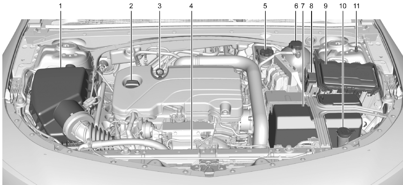
Рядный 4-цилиндровый двигатель с турбонаддувом объемом 1,5 л
