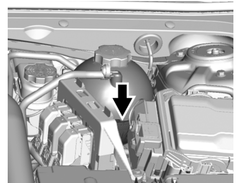
Расширительный бачок охлаждающей жидкости рядного 4-цилиндрового двигателя с турбонаддувом объемом 1,5 л и рядного 4-цилиндрового двигателя с турбонаддувом объемом 2,0 л
